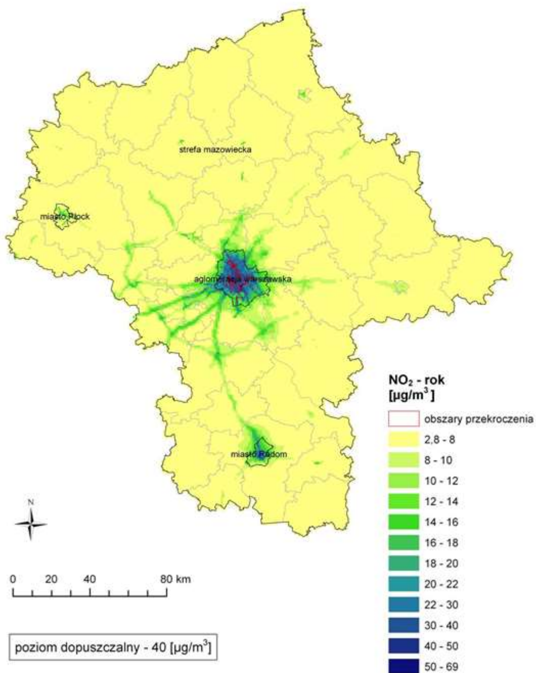
Mapa 2.1. Rozkład stężeń NO 2 -rok na obszarze województwa mazowieckiego (rok 2015) (źródło: WIOŚ w Warszawie)
